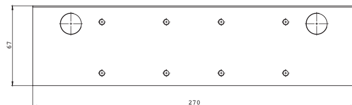
Plaque de montage pour porte vitrée A166
